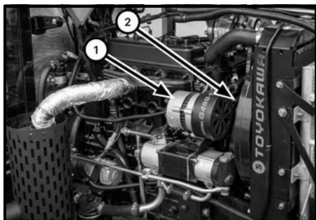
Рис. 5-23. Генератор
