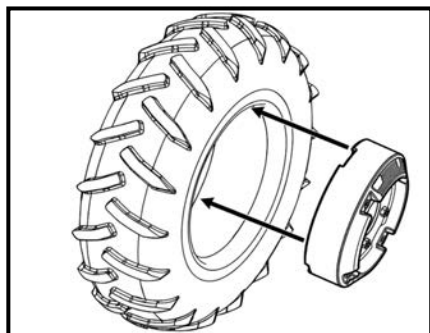
Рис. 4-6. Противовесы на задних колесах
